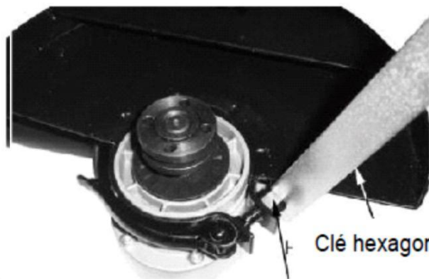
Ecrou hexagonale
