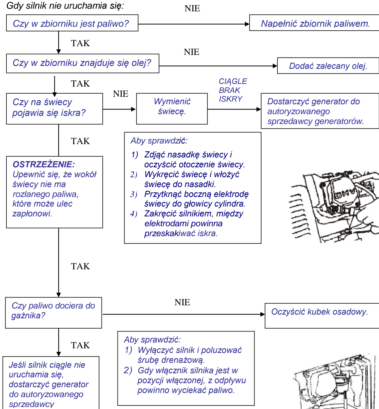
ŚRUBA DRENAŻOWA
