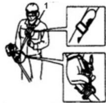
Fig.BC7 1. Strap
