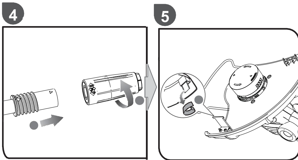
Fig. 5: Retrait de la protection adhésive se trouvant sur le coupe-fil.
